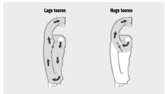
Luchtstroomvariabele inlaatlengte
