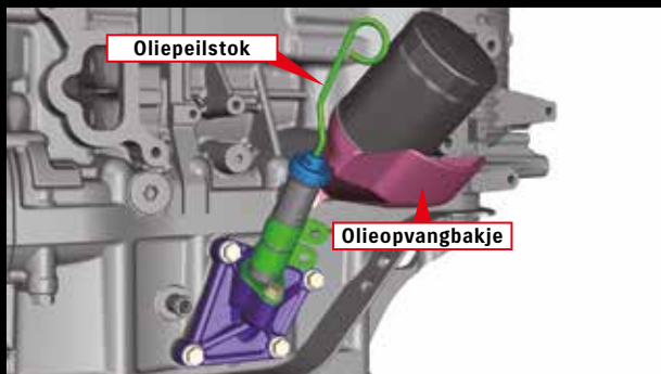
Olieopvangbakje en oliepeilstok
